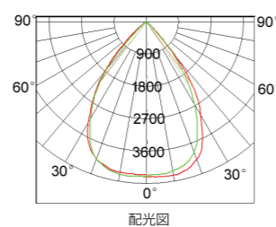
配光図
